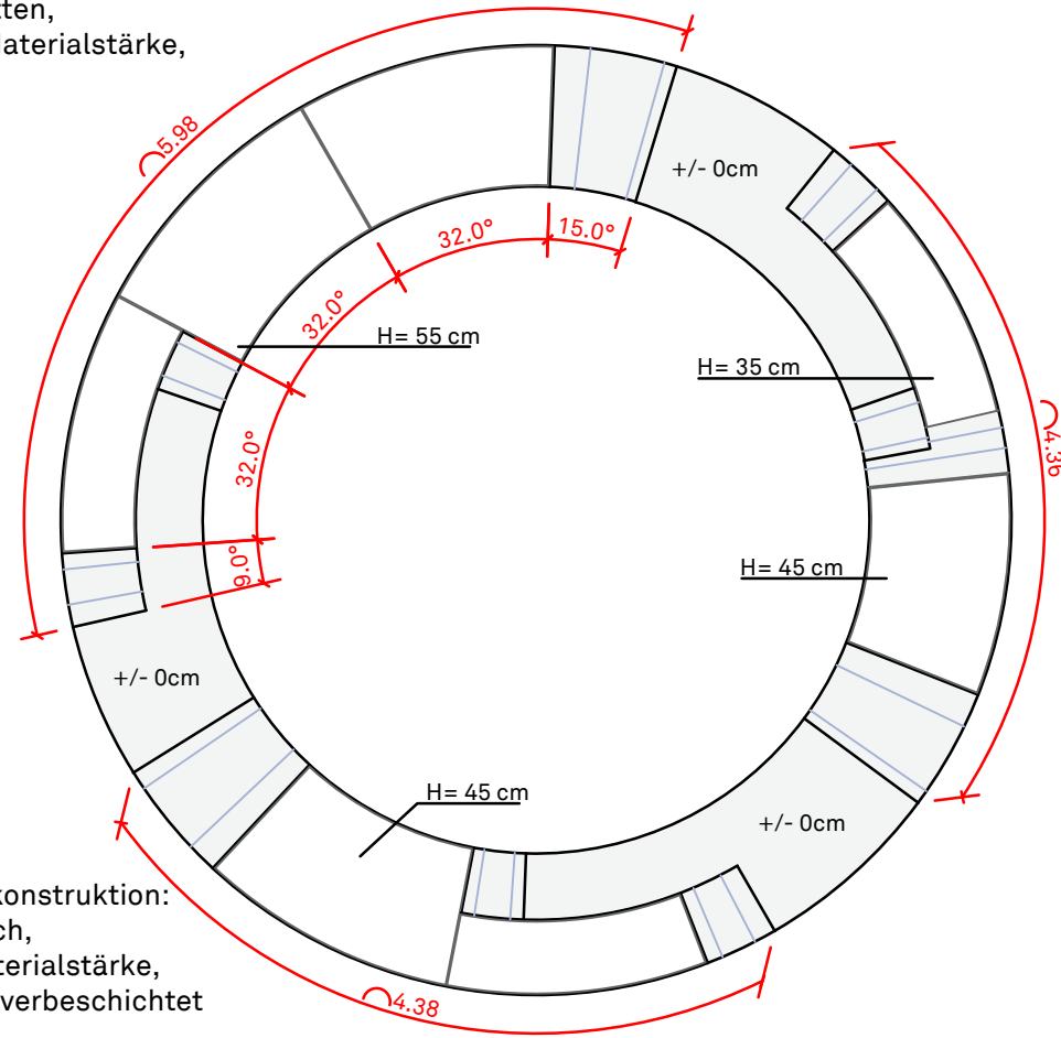
Draufsicht, M 1:50
