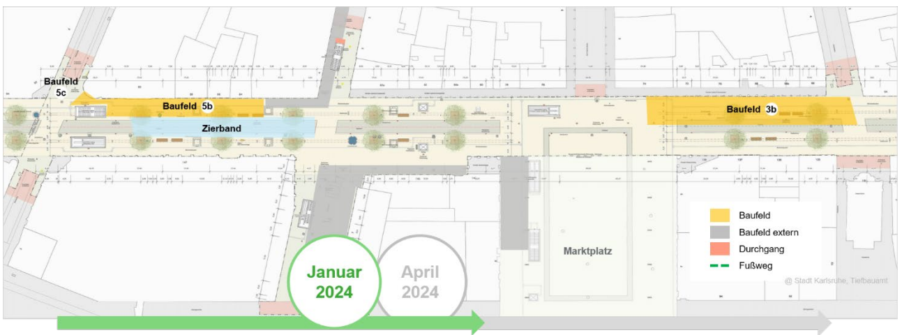
Abbildung 4: Baufelder Januar bis April 2024, Teil 1
