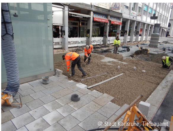
Abbildung 2: Arbeiten um den Aufzug zur Haltestelle
